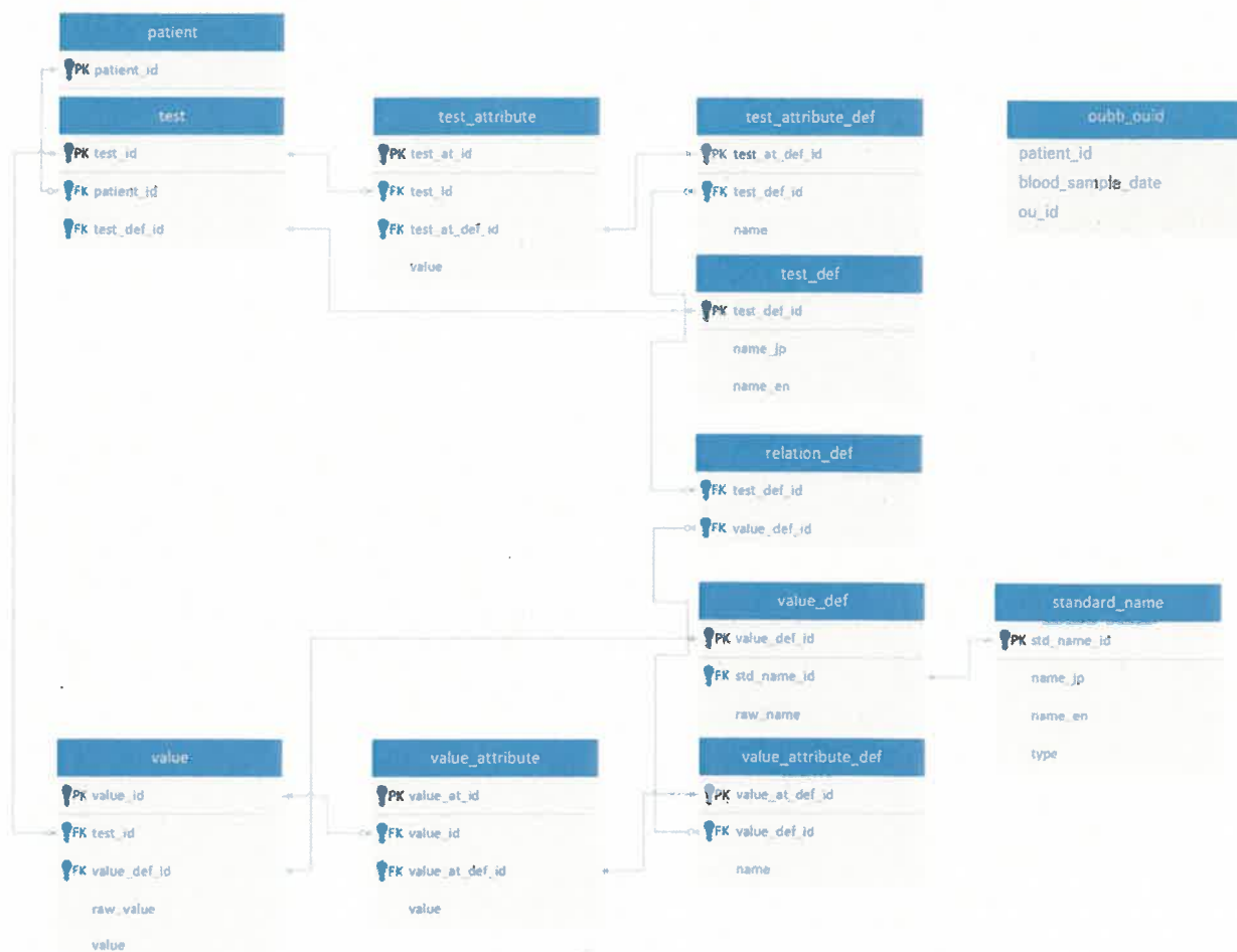
図 2-1 スキーマ
