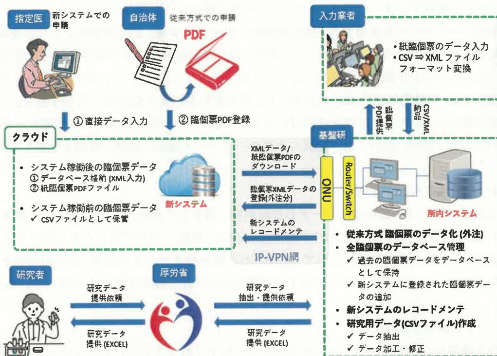
図1 新システム稼働後の業務とシステム構成
